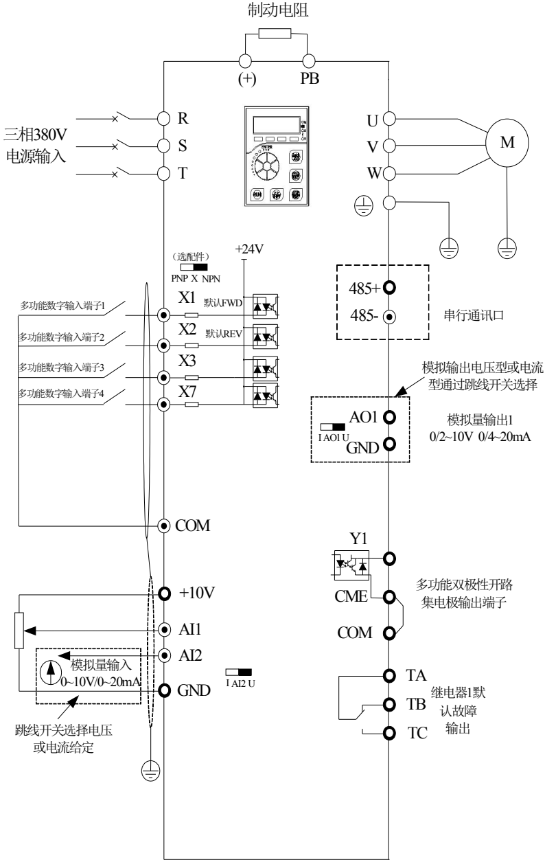
图3-1.2. 2.2kW (4T:380V 2.2 kW) 以下三相变频器接线图
