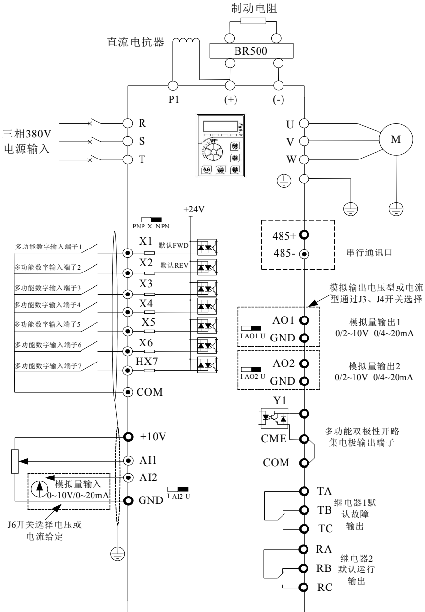
图 3-4. 75Kw (4T: 380V 75 Kw) 及以上三相变频器
