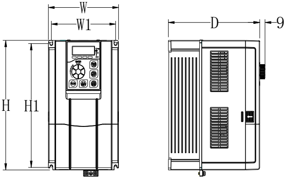
图 2-4. 7.5KW 以下塑胶外形尺寸及安装尺寸示意图
