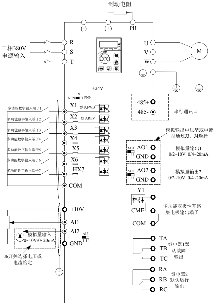
图 3-2. 4.0~ 22kW (4T:380V 4.0 ~ 22kW) 三相变频器接线图
