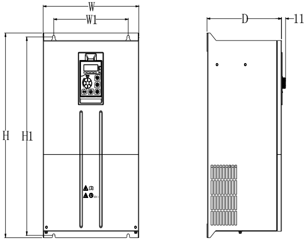
图 2-5. 11~132KW 钣金机箱外形尺寸及安装尺寸示意图
