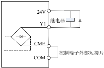
内部供电接线图
