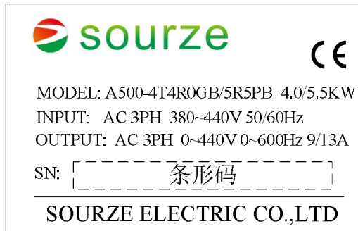
图2-2. 铭牌
