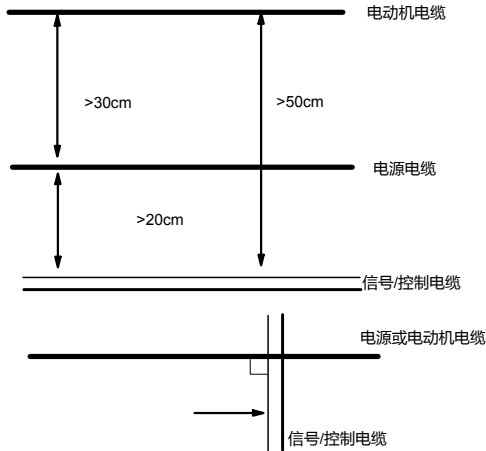
图 4-15 系统配线要求
