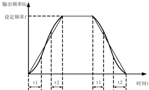
图 6-2 S 曲线加减速方式 1 示意图
