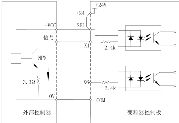
图 4-11 漏型接线方式
