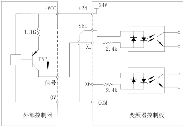
图 4-13 源型接线方式
