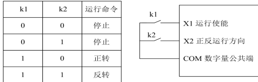
图 6-9 两线式模 2
