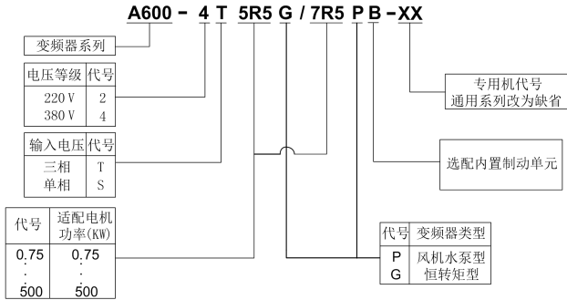
图 3-1 A600 变频器型号
