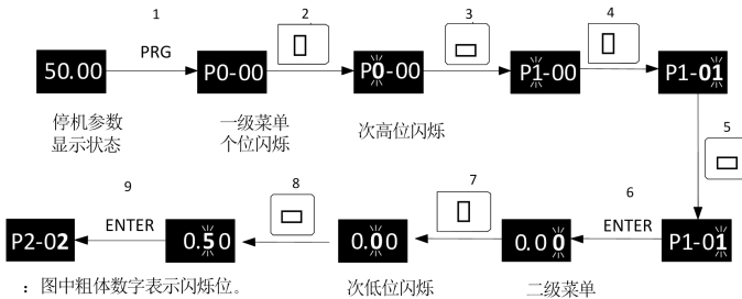
图 5-2 功能码参数设置实例
