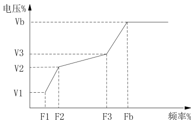
图 6-5 多点 V/F 曲线设定示意图
