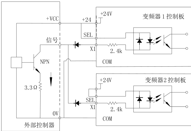
图 4-12 多台变频器 X1 端子并接漏型接线方式
