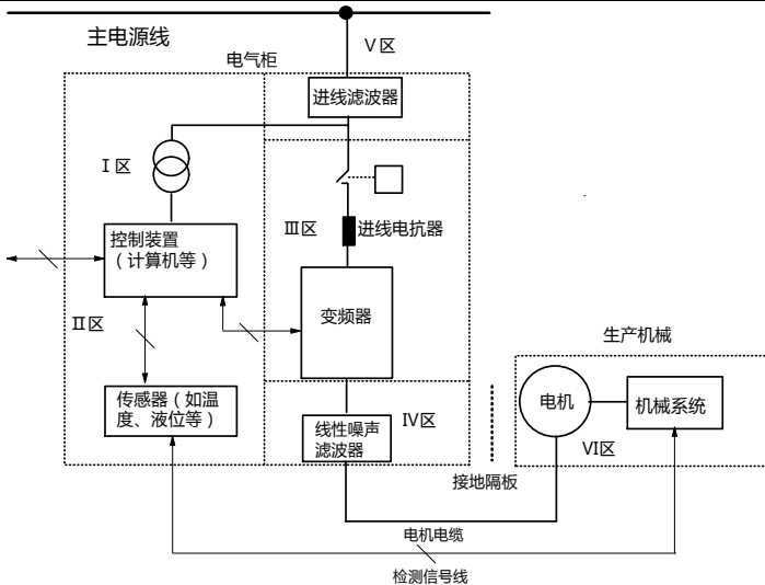
图 4-4 变频器 EMC 安装推荐区域划分示意图
