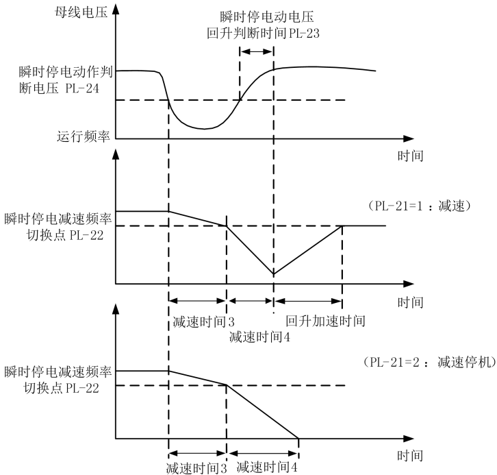
图 6-29 瞬停不停动作示意图
