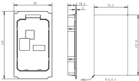
图 3-4 键盘盒的外形及安装尺寸
