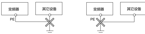
图 4-20 接地示意图 3
