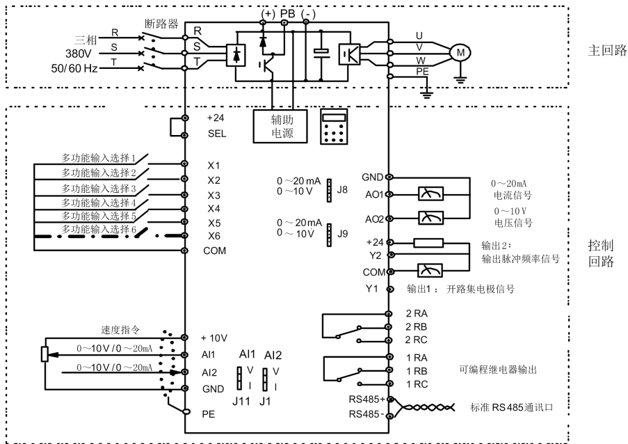
图 4-7 基本配线图
