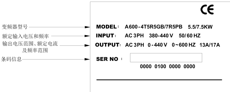
图 3-2 A600 变频器铭牌
