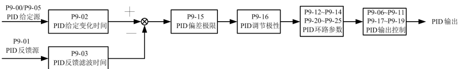
图 6-15 过程 PID 原理框图
