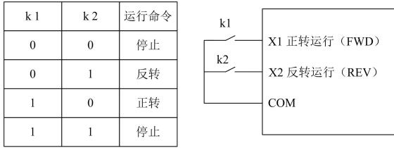
图 6-8 两线式模式 1
