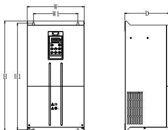
图 2-5. A300(S)系列 15~132KW 钣金机箱外形尺寸及安装尺寸示意图
