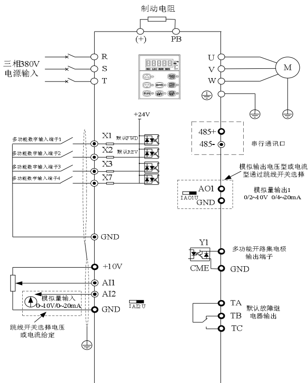
图 3-1. A300(S)系列 2.2kW (4T:380V 2.2 kW) 及单相 220V 2.2kW 以下 220V 接 R T 或 L N, A300N 系列 5.5kW (4T:380V 5.5 kW) 以下三相变频器接线图
