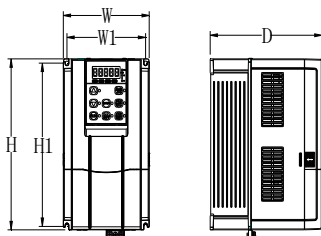
图 2-4. A300(S)系列 11KW 以下塑胶外形尺寸及安装尺寸示意图 (A300N 22KW 以下为塑壳机箱)
