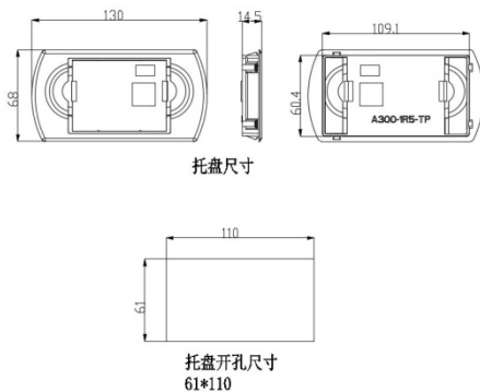
图 2-8.1 小号外引键盘带托盘安装尺寸图 (A300(S)系列 4T:380V 2.2kW 以下标配小号外引键盘, A300N 系列 4T:380V 5.5kW 以下标配小号外引键盘)
