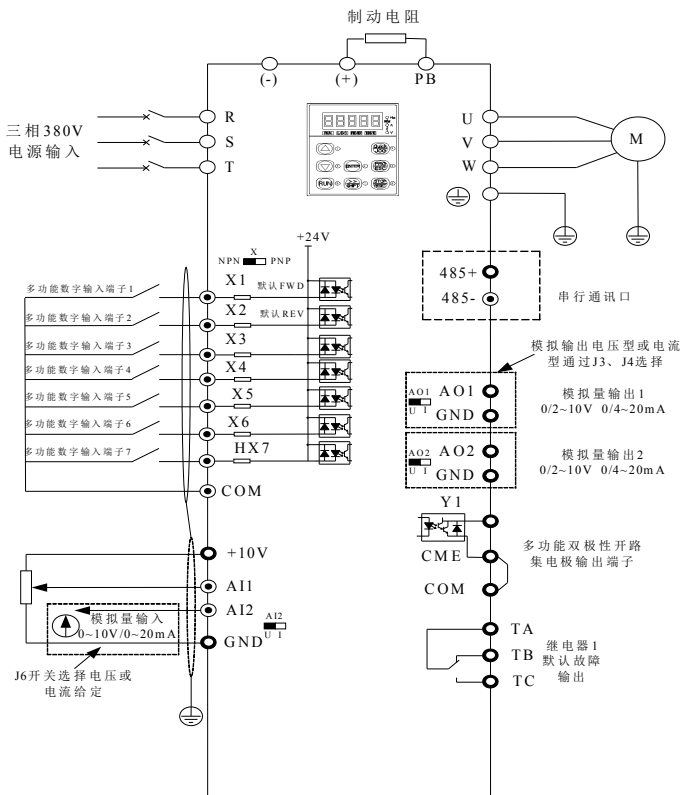
图 3-2. A300(S)系列 4.0~ 30kW (4T:380V 4.0 ~ 30kW), A300N 系列 7.5~ 30kW (4T:380V 7.5 ~ 30kW) 三相变频器接线图
