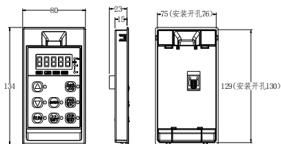
图 2-8.3 大号外引键盘带托盘安装尺寸图 (A300(S)系列 4T:380V 55kW 以上标配大号外引键盘, A300N 系列 4T:380V 15~22Kw, 55Kw 以上标配大号外引键盘)
