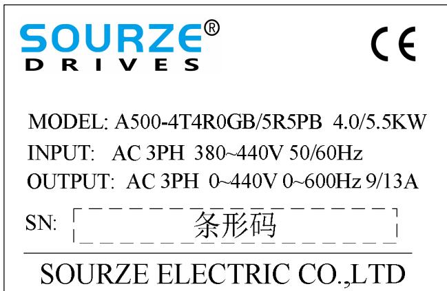
图2-2. 铭牌
