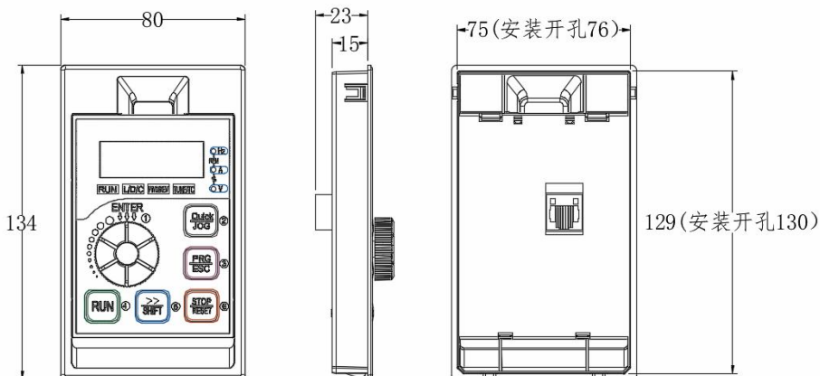
图 2-8.2 大外引键盘带托盘安装尺寸图 (4T:380V 45kW以上标配大外引键盘)
