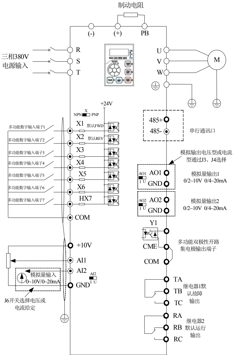
图 3-2. 三相 380V 4.0~ 22kW (4T:380V) 及单相 220V (3S) 5.5kW 以下(输入接 R T)变频器接线图 备注: 数字输入端子 X 跳线开关出厂默认 NPN 模式 (即 X 短接 COM 有效), AI2, AO1, AO2 跳线开关出厂默认电压模式
