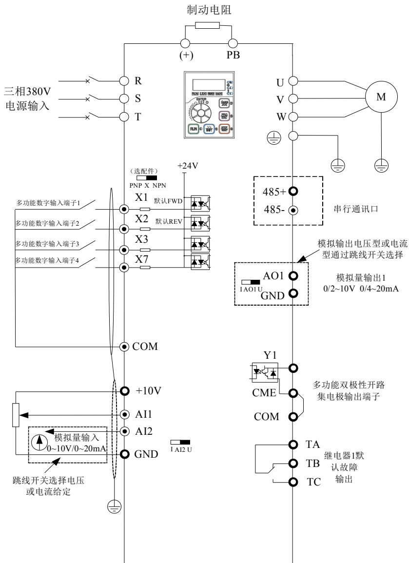
图3-1. 三相380V 2.2kW (4T:380V) 及单相220V (3S) 1.5kW(输入接L N或R T)以下变频器接线图
