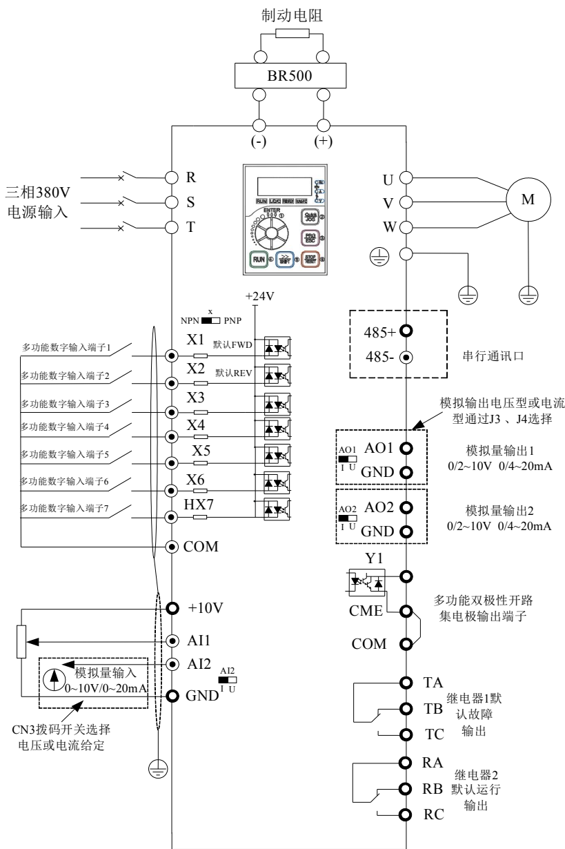
图 3-3. 三相 380V 30 ~ 55 kW (4T:380V) 变频器不带制动单元功能接线图
