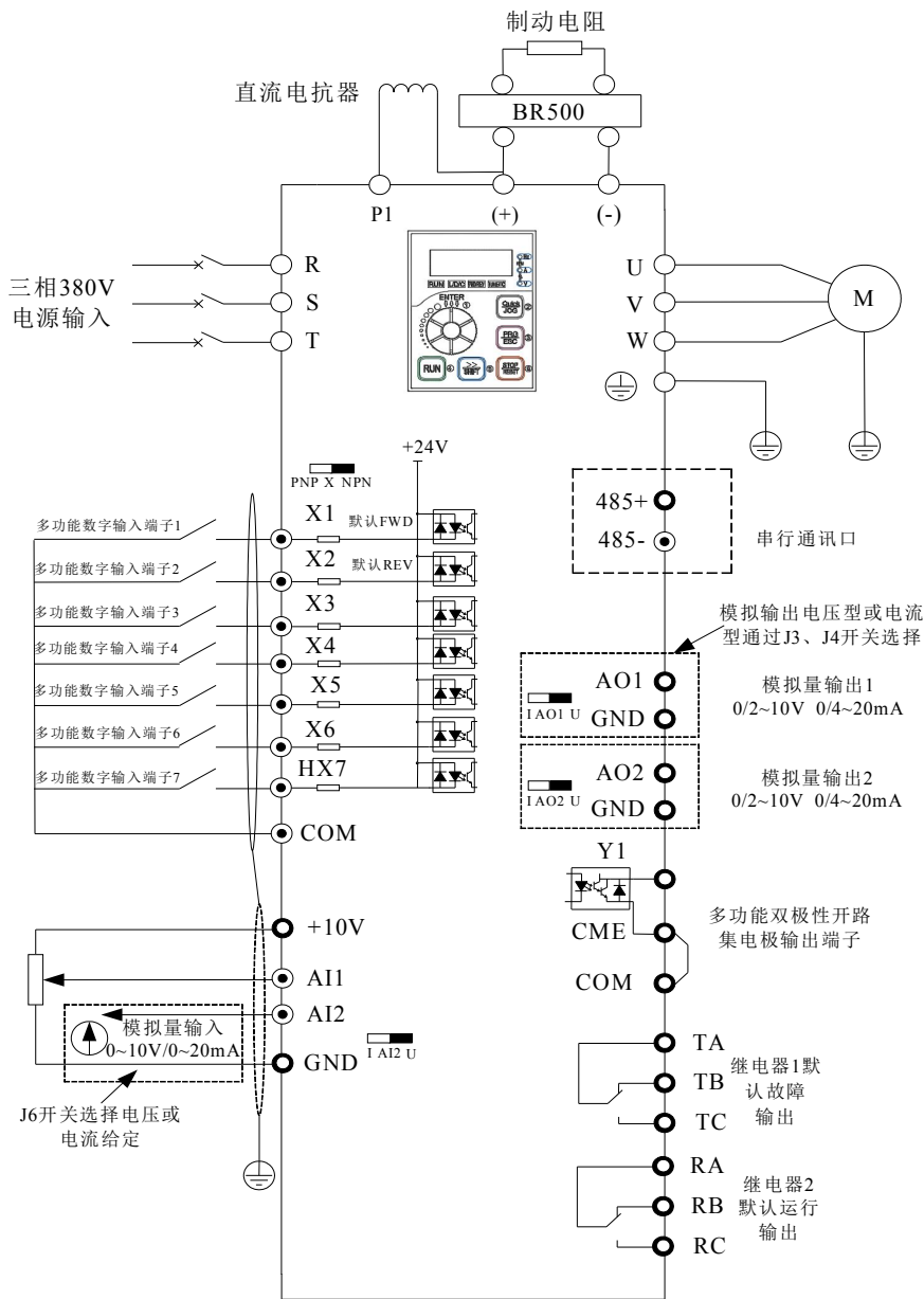
图 3-4. 三相 380V 75kW (4T:380V) 及以上三相变频器接线图
