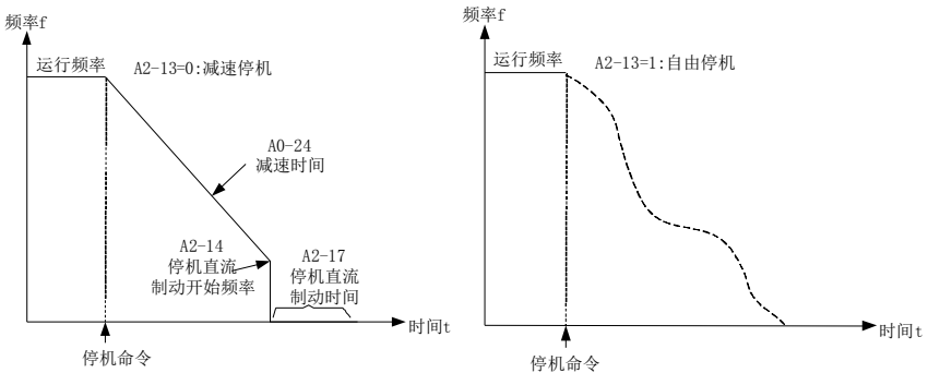
图4-13. 停机示意图
