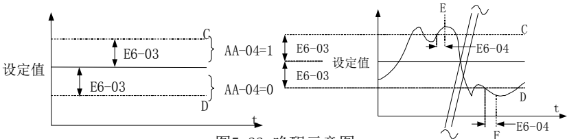
图5-33. 唤醒示意图
