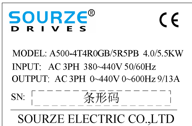
图2-2. 铭牌
