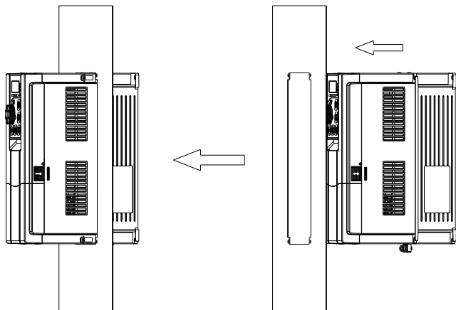
图3-3. A500/A500S变频器塑胶结构穿墙式安装图
