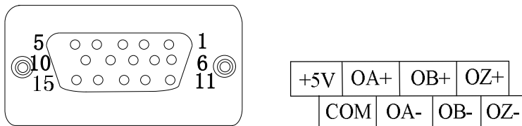
附录 B: 图 7 A700-PGS 端子图
