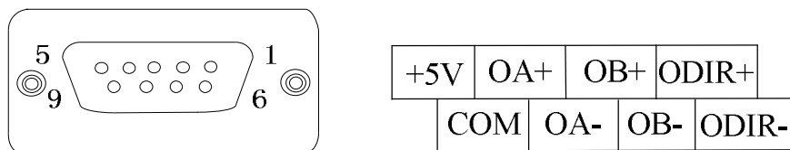
附录 B: 图 5 A700-PGR 端子图
